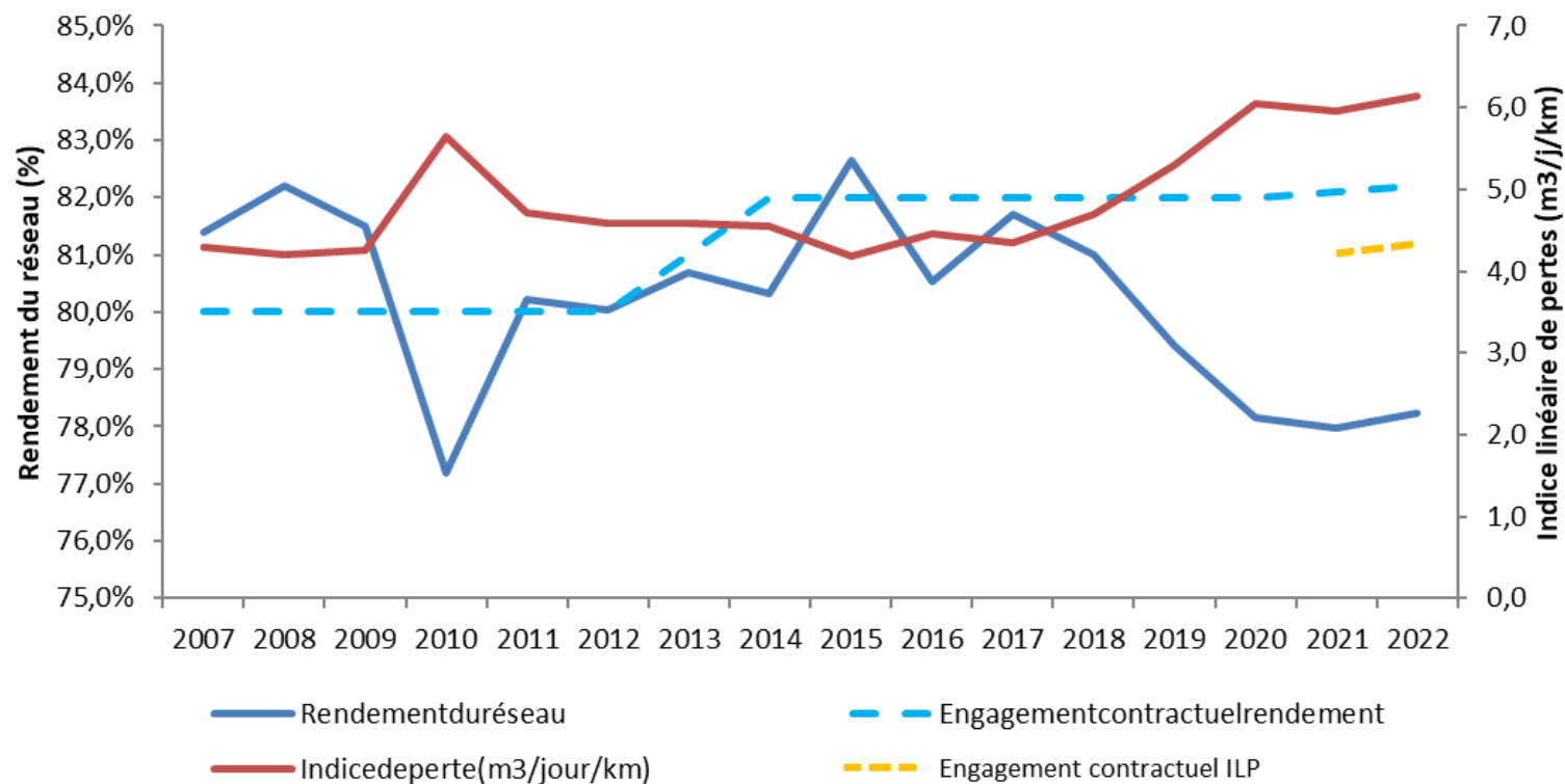
Evolution du rendement et des pertes en réseau
